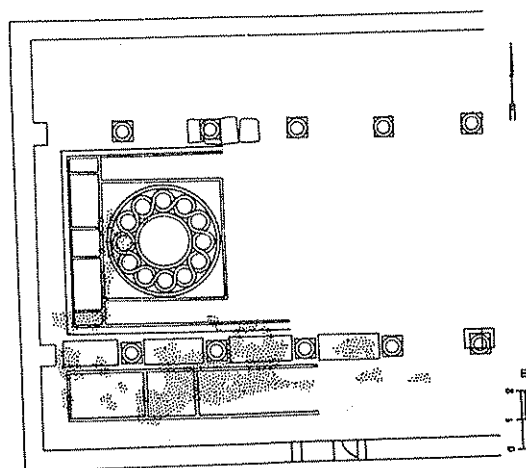
תכנית בית הכנסת ביפיע
