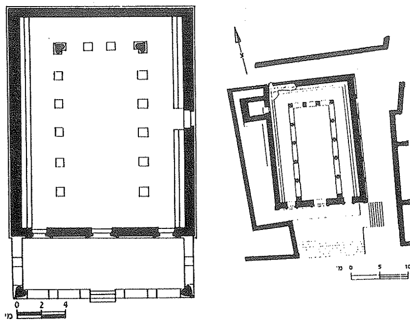
כורזים: תכנית בית הכנסת
